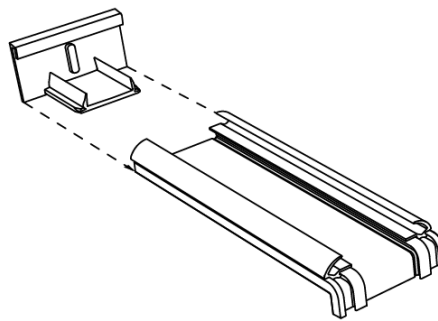
Unsichtbare Verbindungsplatte
